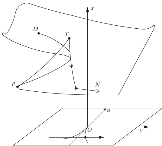
图 1 尖点突变的平衡曲面和分叉集
