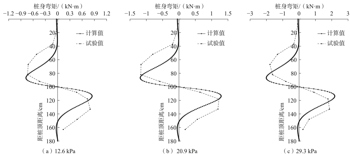
图 9 不同加载应力下后排桩桩身弯矩
