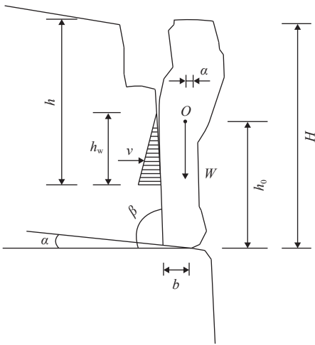
图 12 稳定性计算模式示意图 Fig. 12 Stability calculation mode
