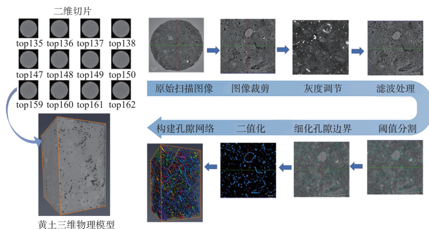
图 2 CT 图像处理流程图
