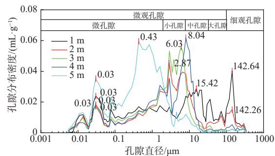
图 3 孔隙密度分布曲线 Fig. 3 Pore density distribution curve
