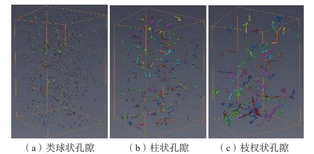
图 9 基于三维形状因子的黄土孔隙分类
