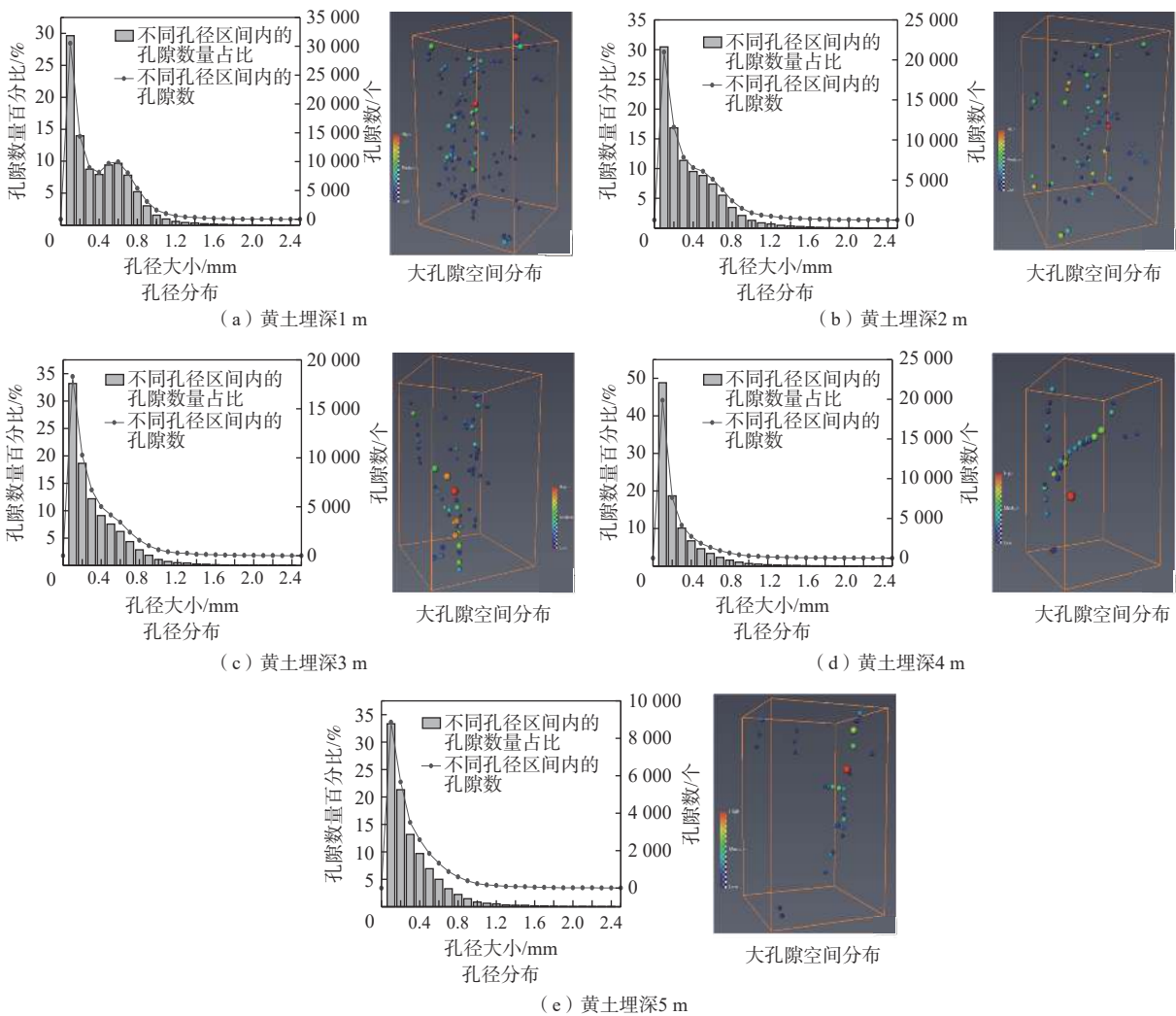
图 7 不同深度黄土的孔径分布图与大孔隙空间分布图
