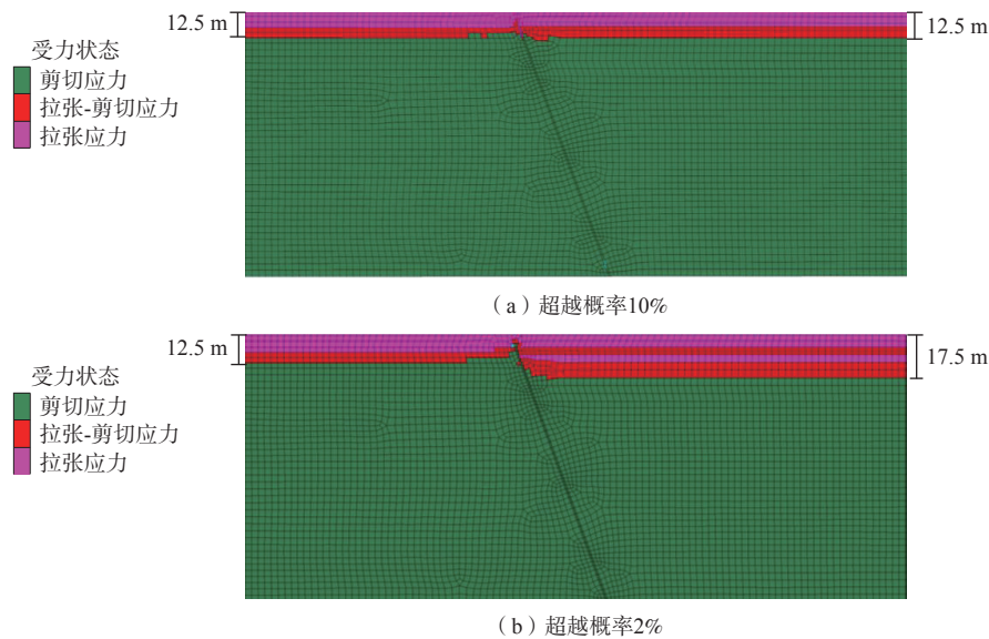
图 17 不同超越概率地震作用下断裂带场地塑性区
