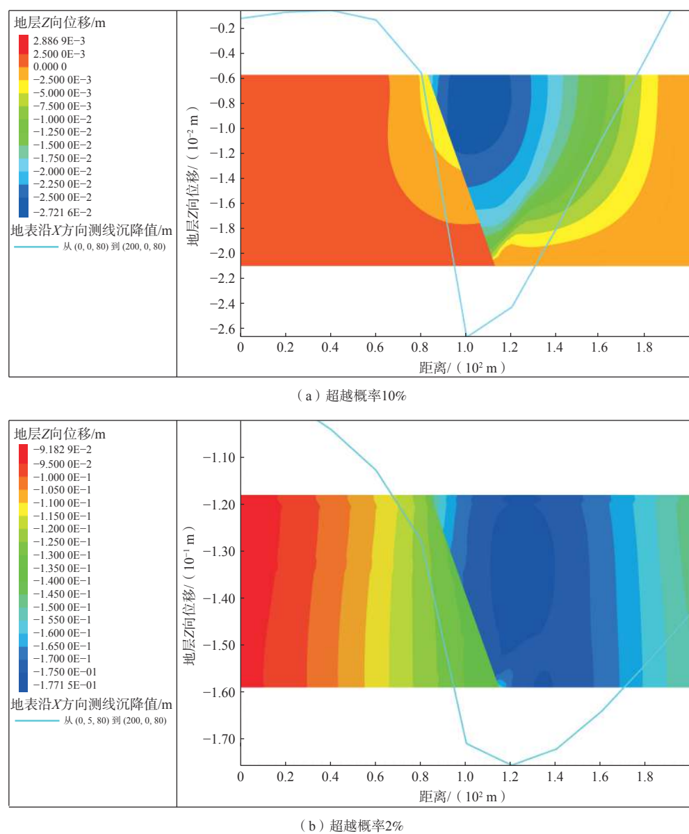
图 15 不同超越概率地震作用断裂带场地竖向位移云图
