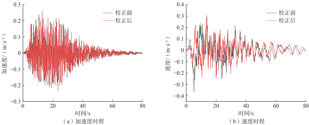
图 7 100 年超越概率 10% 的西安人工地震波
