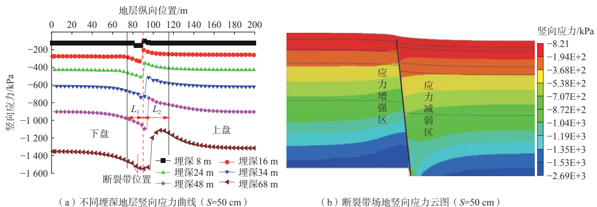
图 9 断裂场地竖向应力特征
