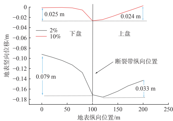
图 16 地表最大竖向位移与纵轴位置关系曲线图
