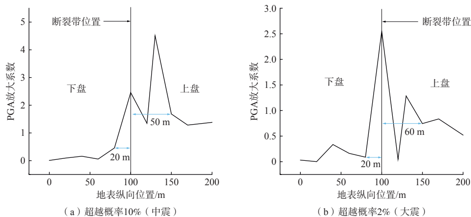
图 18 不同超越概率地震作用下 PGA 放大系数曲线图
