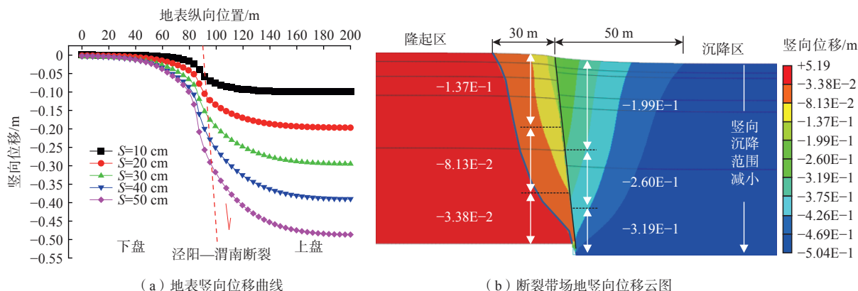
图 11 断裂场地竖向位移特征
