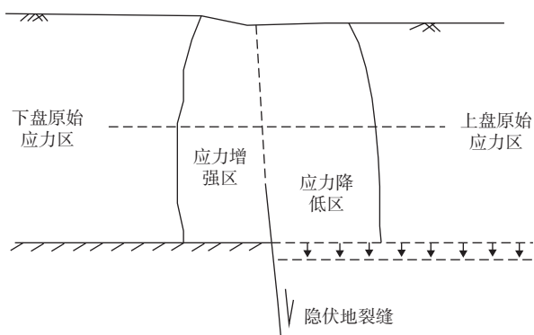
图 10 西安地裂缝错动引起地层应力分布模式 [29]
