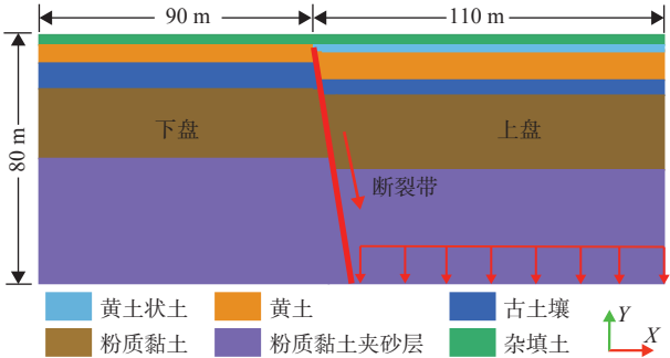
图 4 泾阳—渭南断裂场地同震位错计算模型 Fig. 4 Calculation model of Jingyang-Weinan fault site
