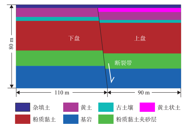
图 5 断裂带场地黏滑动力学计算模型 Fig. 5 Calculation model of fault zone site
