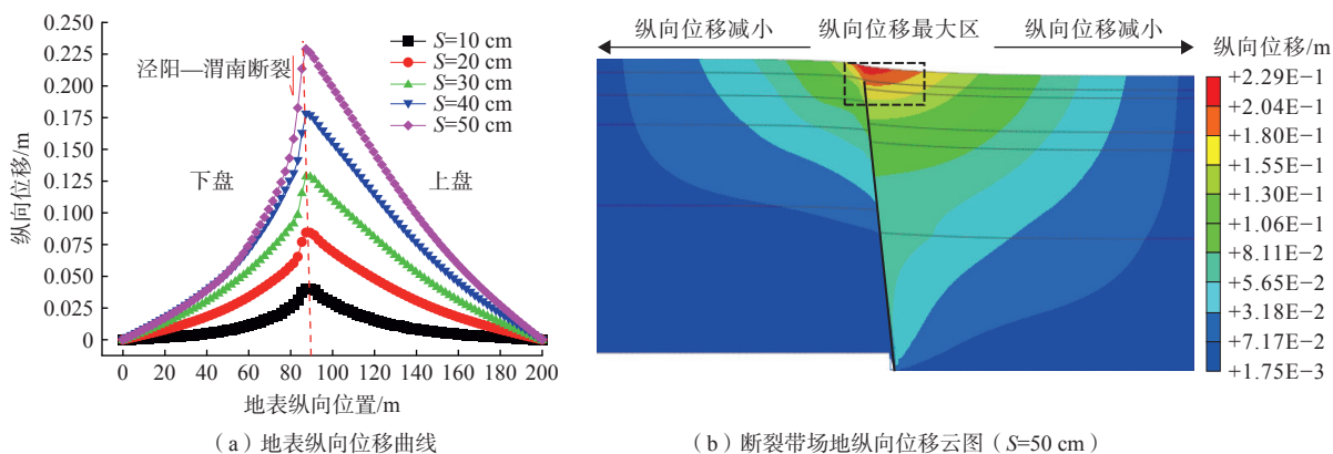
图 12 断裂场地纵向位移特征
