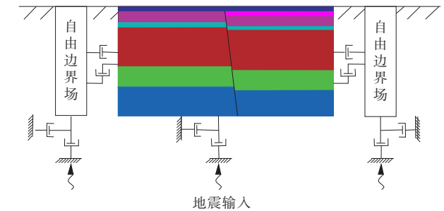
图 6 自由场边界示意图
