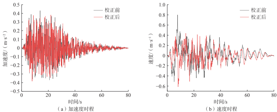
图 8 100 年超越概率 2% 的西安人工地震波
