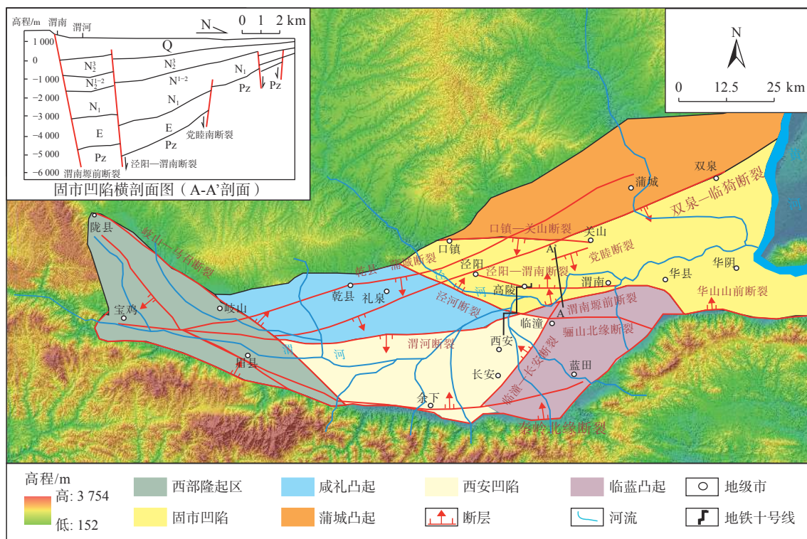
图 1 渭河盆地区域构造图
