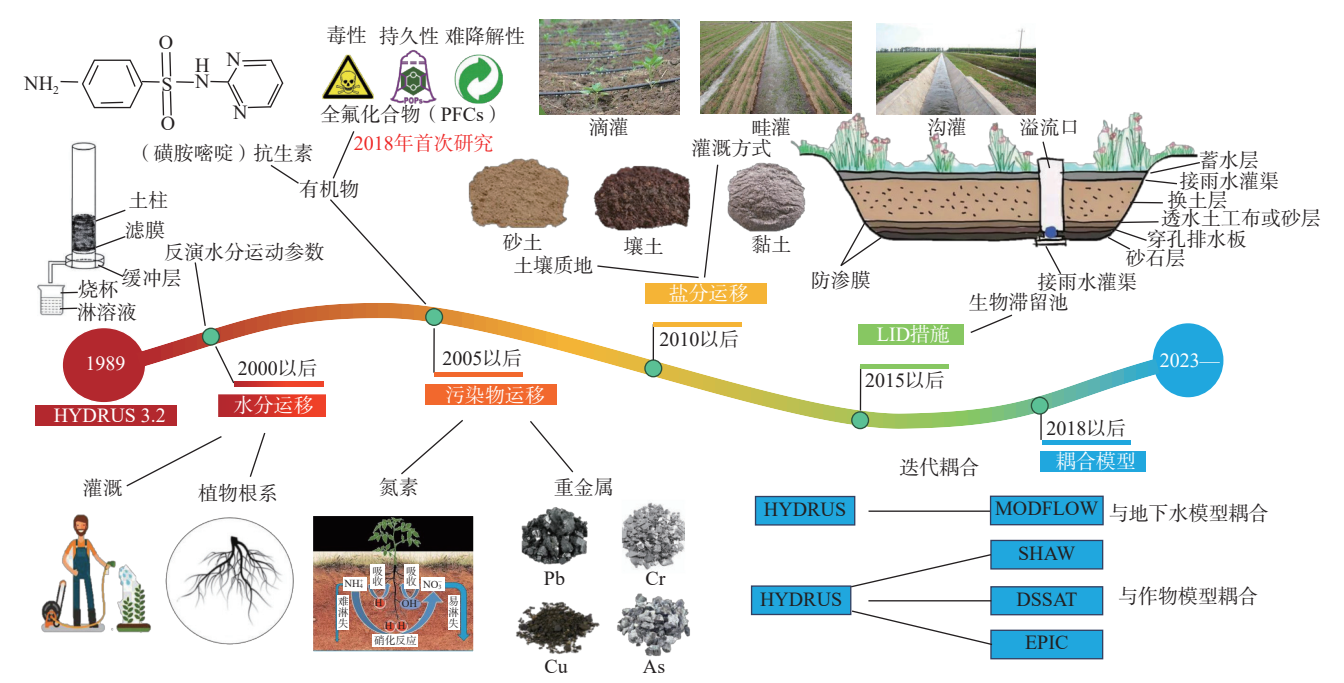
图 2 HYDRUS 模型研究历程 Fig. 2 Research course of HYDRUS model
