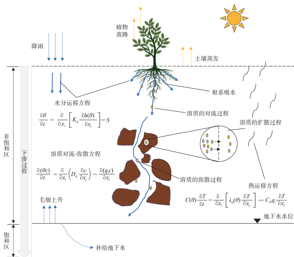
图 1 HYDRUS 模型模拟原理
